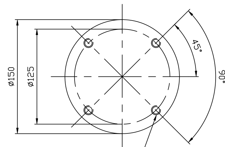
ISO 5211 F12 Vue A de la bride View A of the flange
